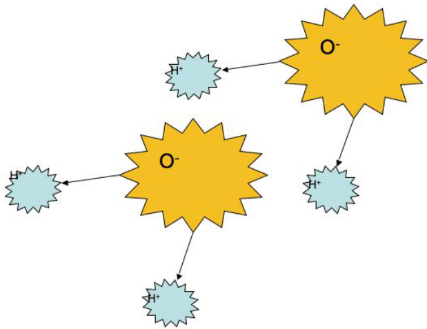
Imbrication des atomes de l'eau en agrégats de 400 molécules
